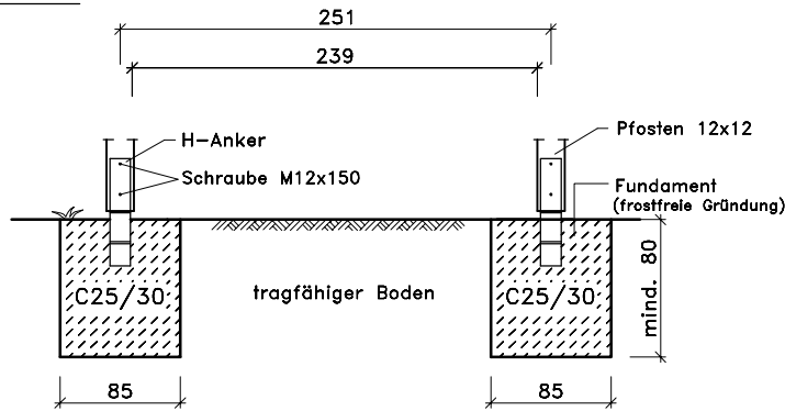
Schnitt B-B
