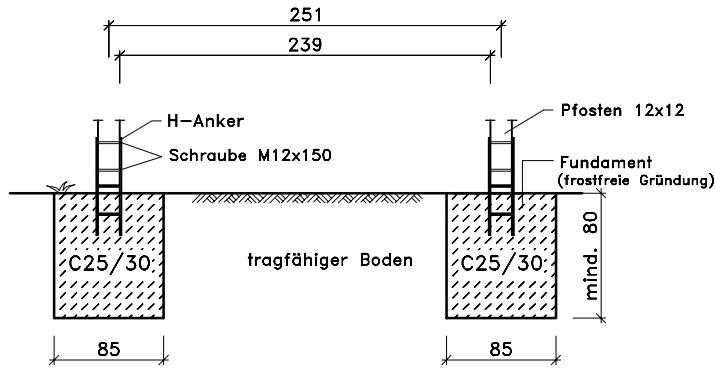
Schnitt A-A
